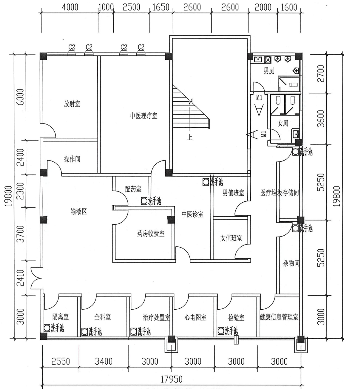
医务室装修平面图
